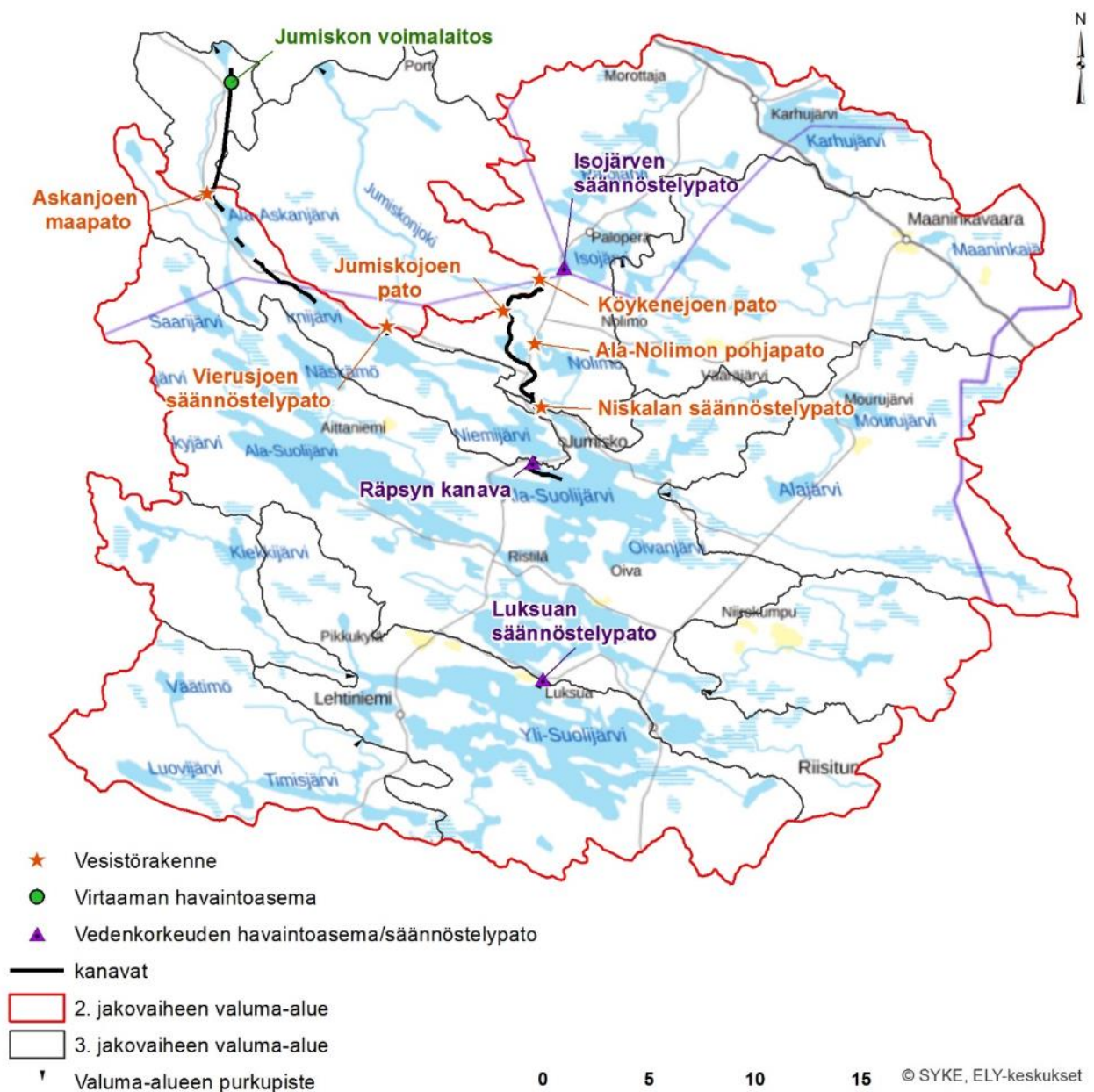
Kuva 1. Jumiskon voimalaitoksen vaikutusalueen säännöstelykokonaisuus.
