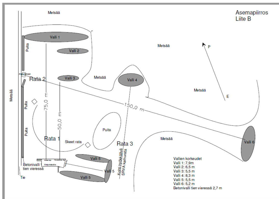
Kuva 1. Asemapiirros
