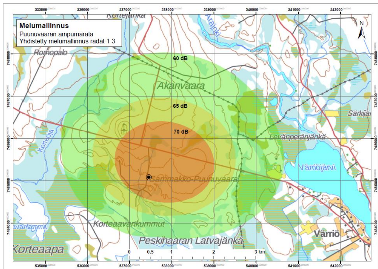
Kuva. 2 Melumallinnuskartta
